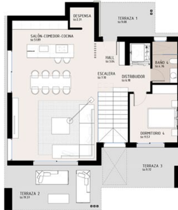
PLANTA BAJA
