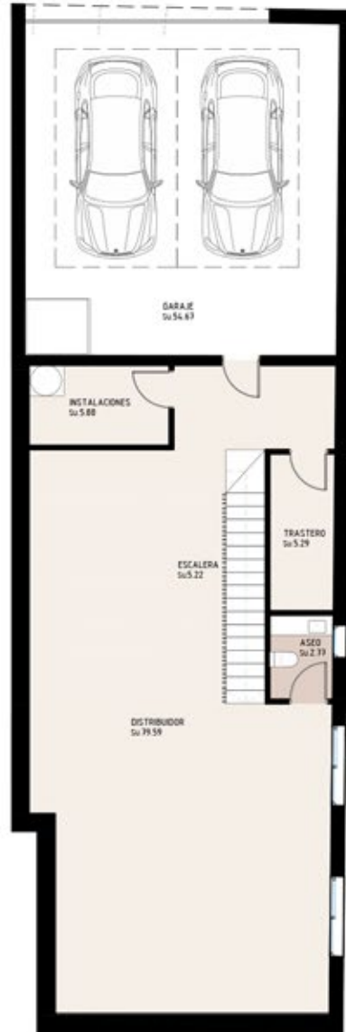
PLANTA SÓTANO
