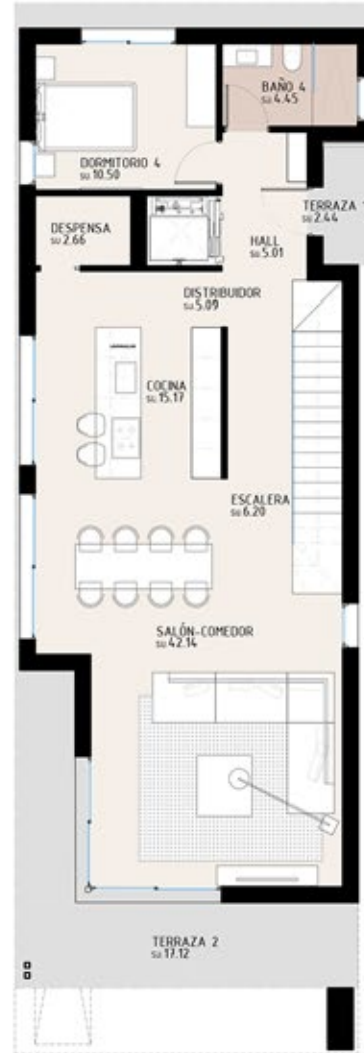
PLANTA BAJA
